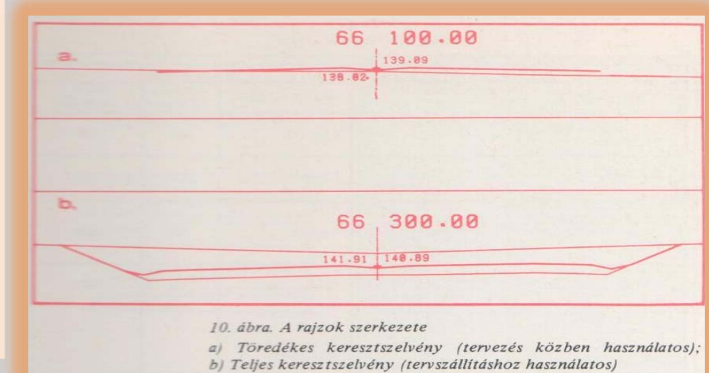
KERESZTSZELVÉNY
